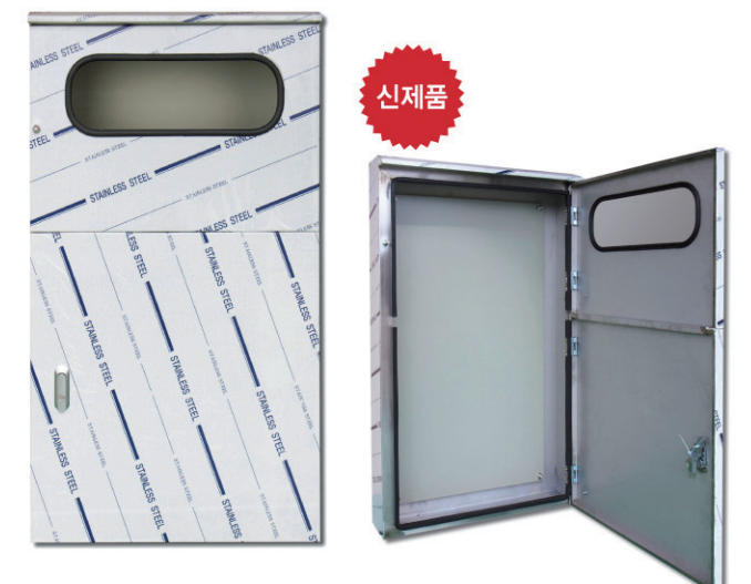
스텐 옥외 SCT 3상 계량기(STS 201, 1.2T)
